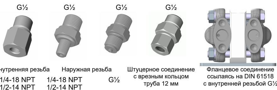
Рис. 2: Параметры для технических подключений
