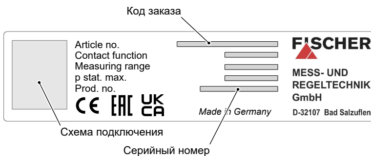
Рис. 3: Заводская табличка
