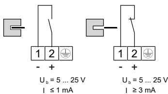
Рис. 16: Индуктивный контакт
