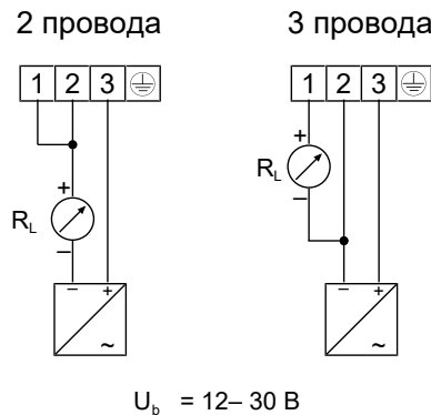
Рис. 17: Подключение — Датчик угла поворота
