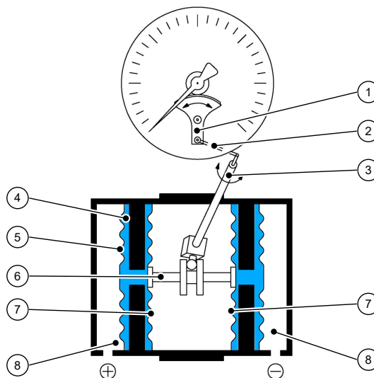
Рис. 11: Функциональная схема
