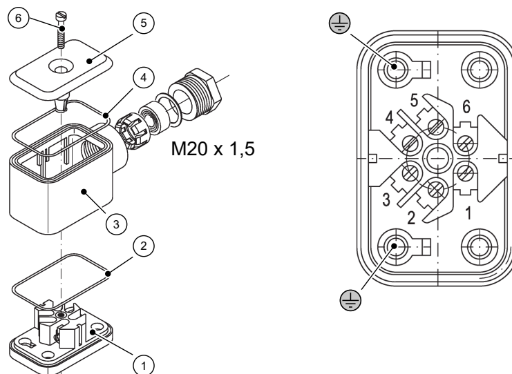
Рис. 13: Кабельная коробка
