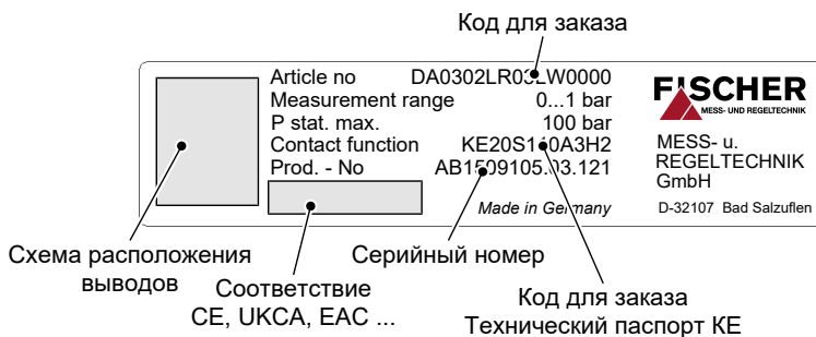
Рис. 3: Заводская табличка
