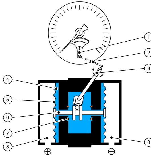
Рис. 7: Функциональная схема
