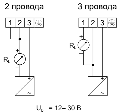
Рис. 13: Подключение — Датчик угла поворота
