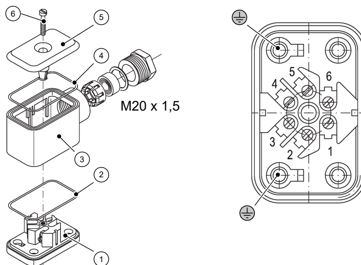
Рис. 9: Кабельная коробка
