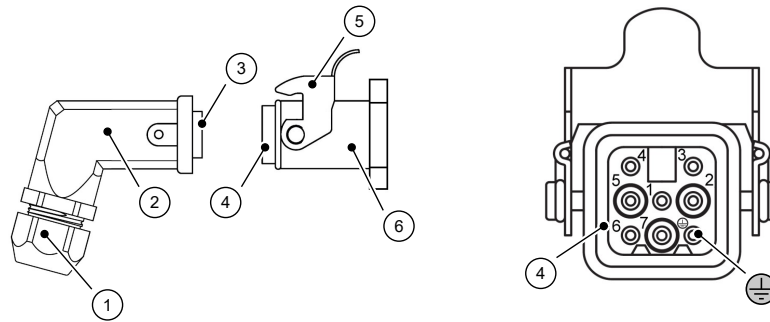
Рис. 10: Штекер HAN
