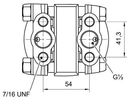
Рис. 19: Схема установки (малая измерительная система Ø 75)
