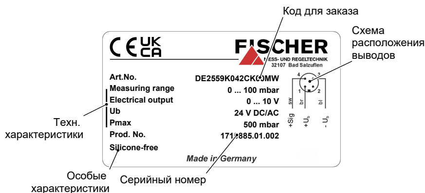
Рис. 2: Паспортная табличка
