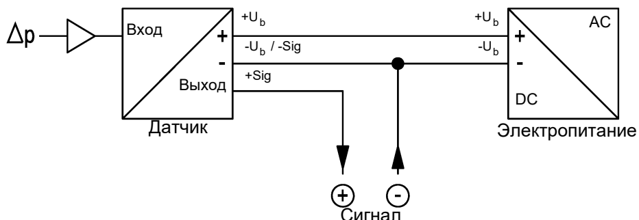
Рис. 5: Трехпроводная схема
