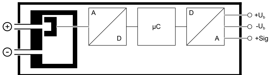
Рис. 3: Функциональная схема
