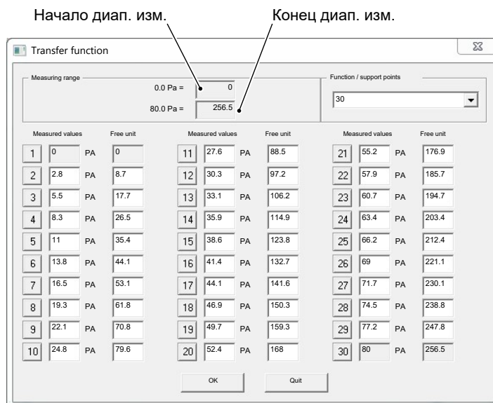
Рис. 14: Функция передачи
