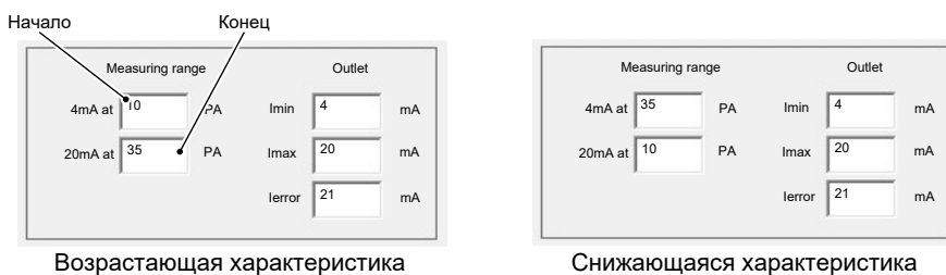
Рис. 11: Характеристическая кривая
