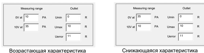
Рис. 12: Характеристика выхода напряжения
