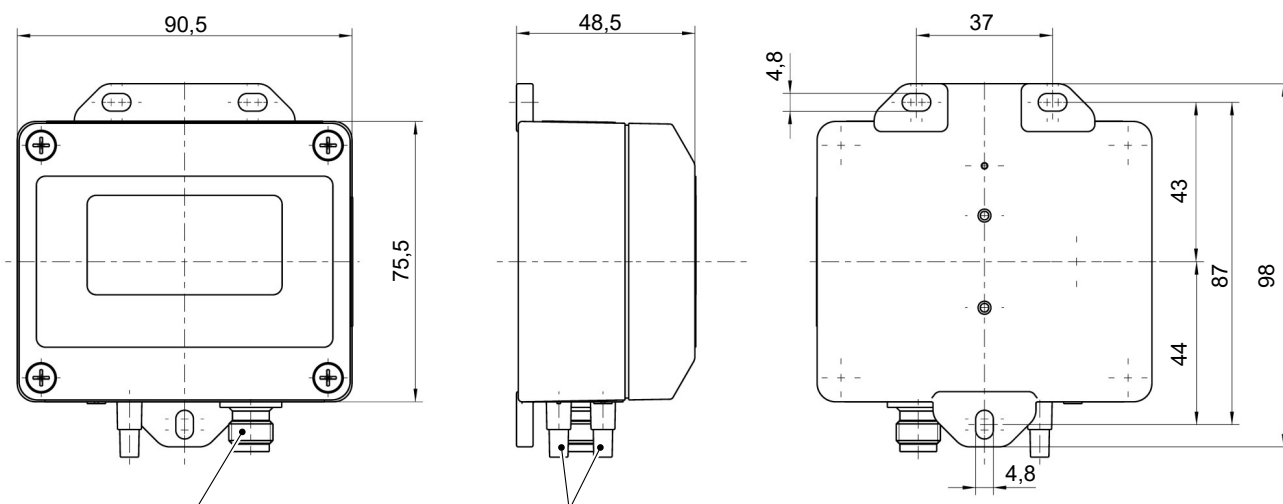
Рис. 16: Габаритный чертёж
