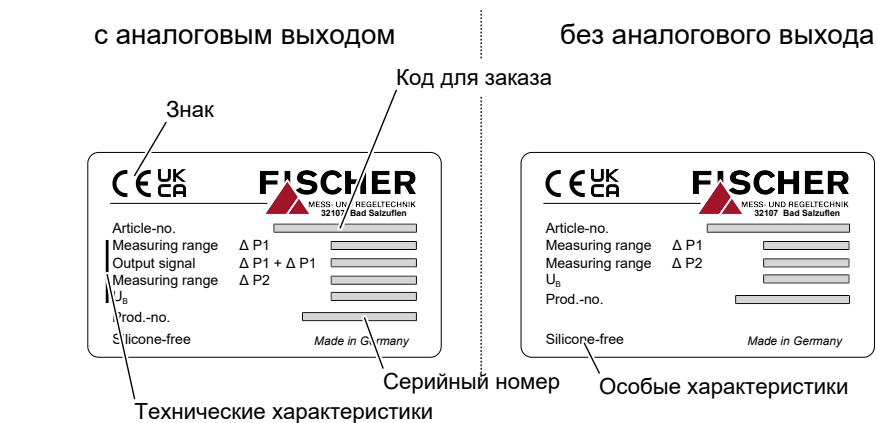
Рис. 4: Паспортная табличка
