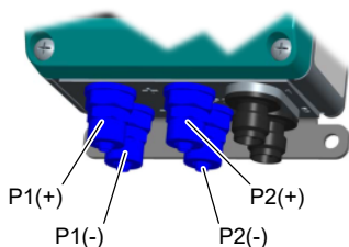
Рис. 5: Техническое подключение
