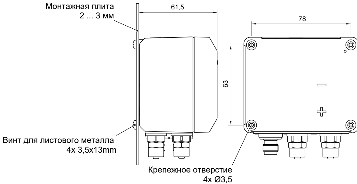
Рис. 27: Чертеж монтажной платы
