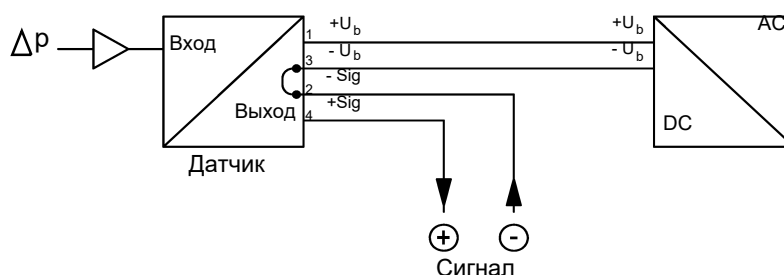
Рис. 4: Трехпроводное подключение с внутренним мостом -U_b / -Sig
