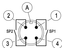
Рис. 6: M12, штекер 4-контактный + выходные контакты
