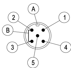
Рис. 5: M12, штекер 5-контактный + мост
