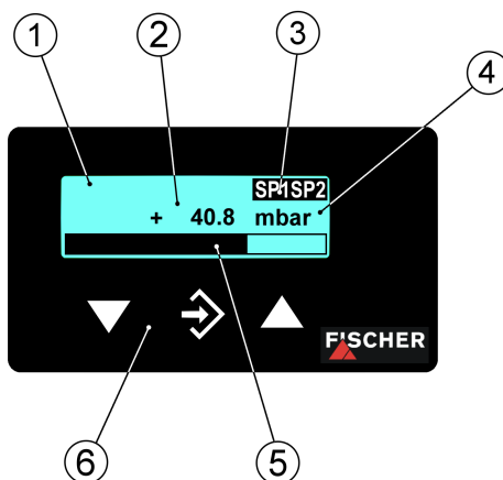
Рис. 7: ЖК-дисплей DE45
