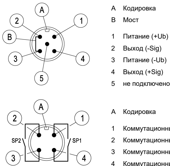
Рис. 17: Электроподключение DE45_LCD
