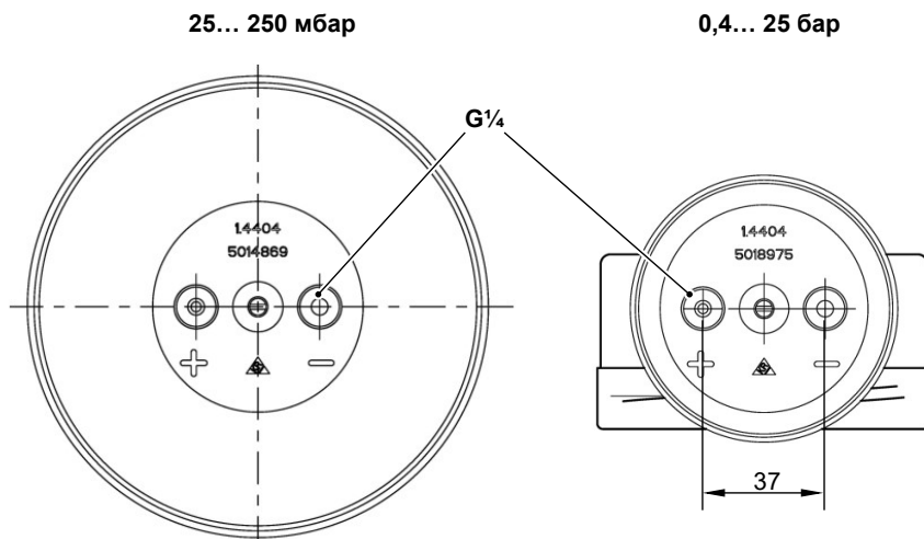
Рис. 7: Техническое подключение
