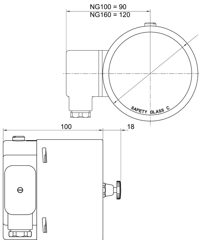
Рис. 12: Корпус с байонетным кольцом и кабельной коробкой
