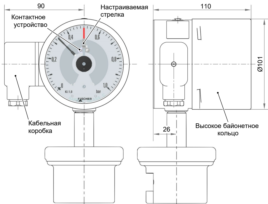
Рис. 11: Защитный кожух
