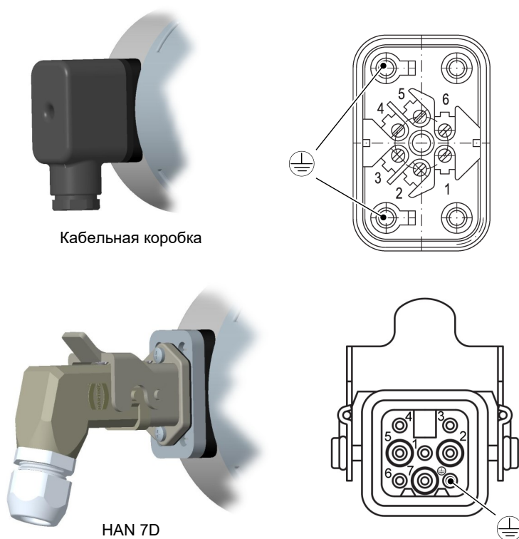
Рис. 4: Кабельная коробка
