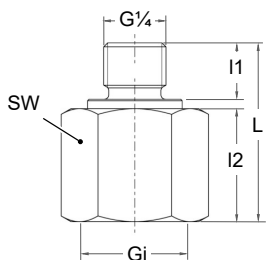
Рис. 10: Соединительная цапфа Gi
