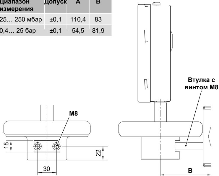
Настенный монтаж
