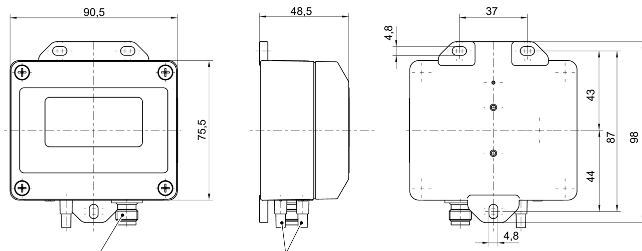
Рис. 4: Габаритный чертеж
