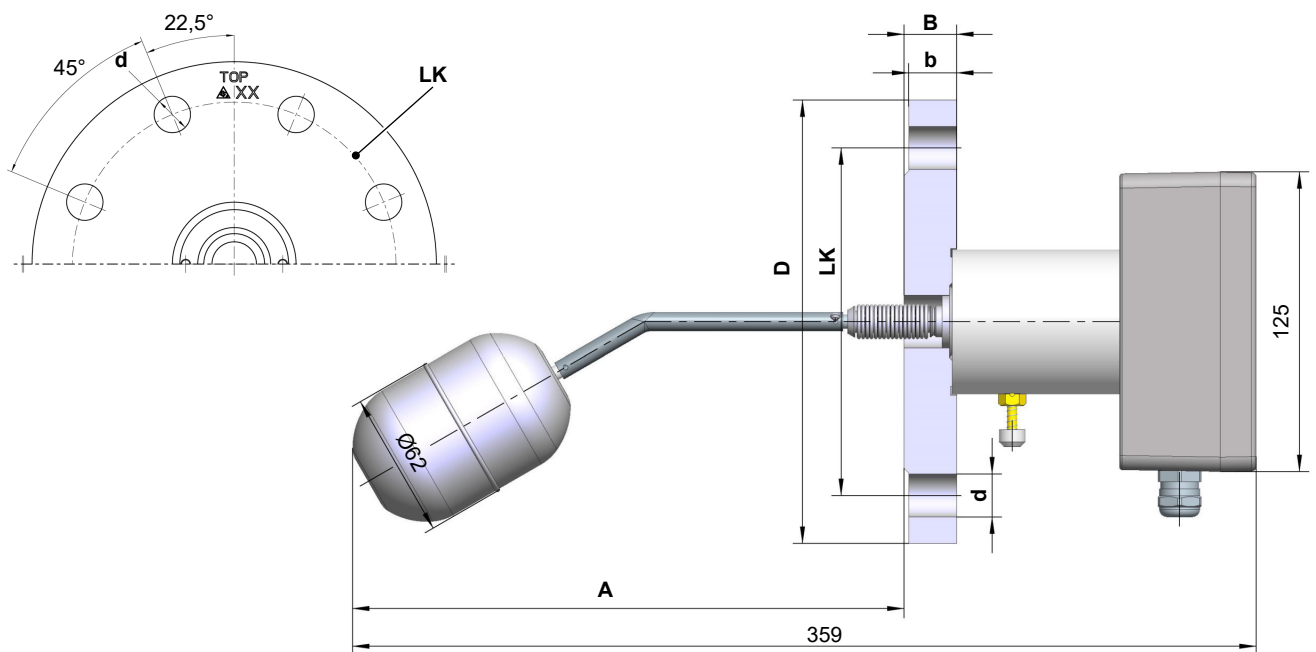
Рис. 10: Чертеж NK10M
