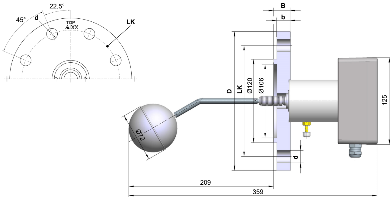
Рис. 5: Чертеж NK10F
