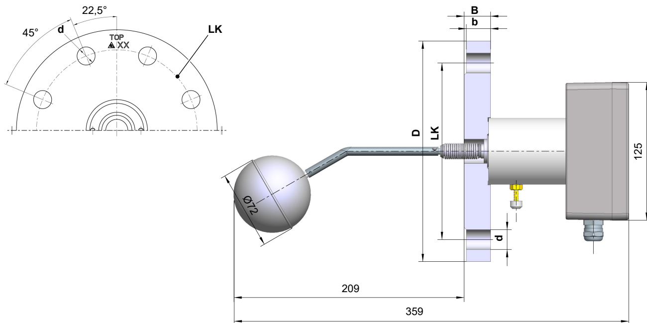
Рис. 3: Чертеж NK102 NK10G
