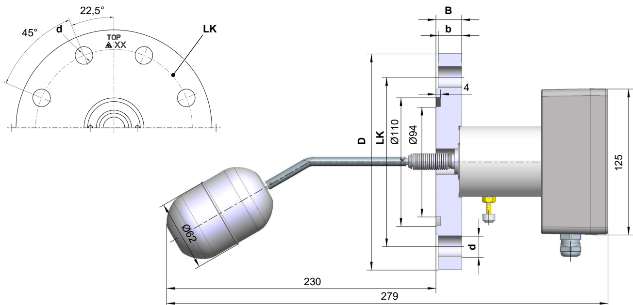
Рис. 8: Чертеж NK10B
