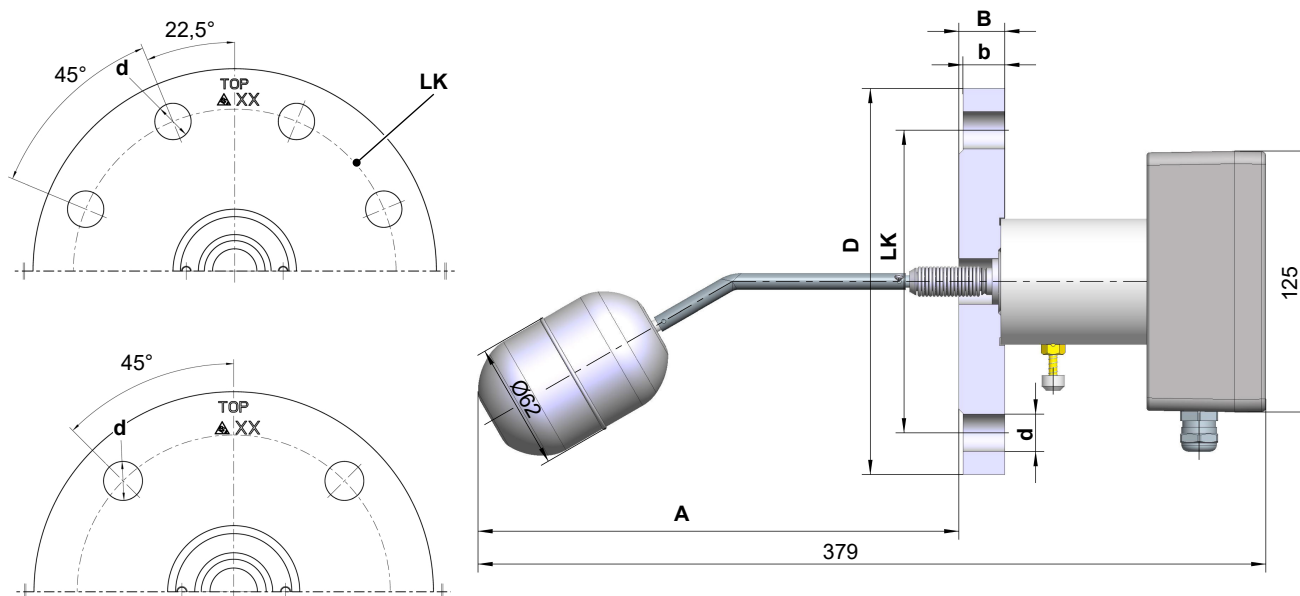
Рис. 4: Чертеж NK101 NK103 NK107
