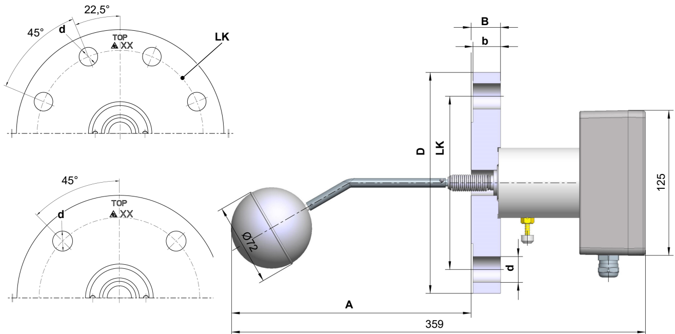
Рис. 9: Чертеж NK10K NK10N NK10P
