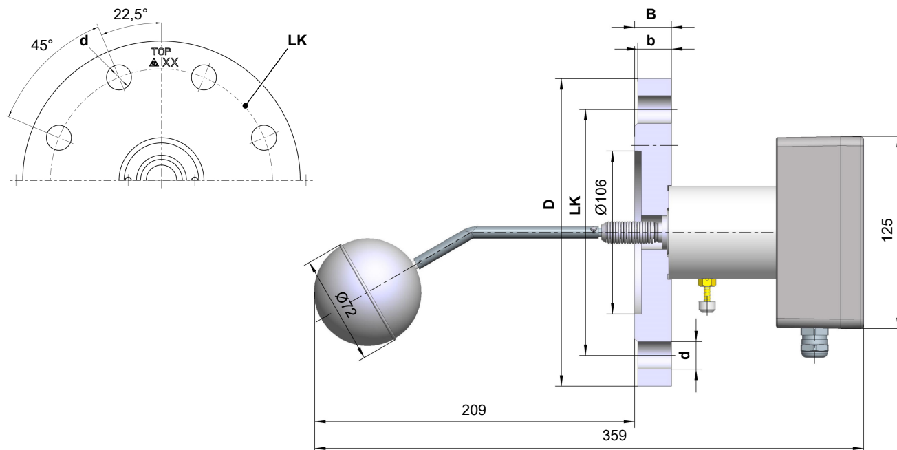
Рис. 7: Чертеж NK10H
