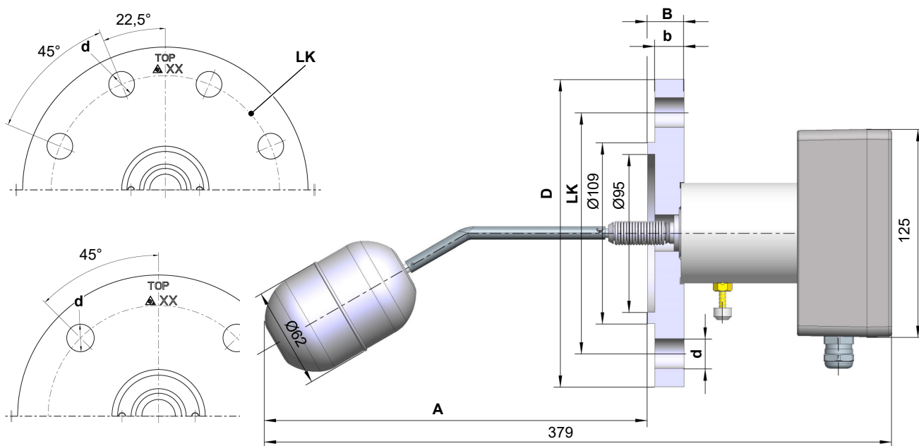
Рис. 6: Чертеж NK106 NK10A
