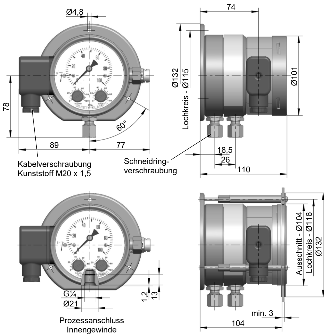
Abb. 9: Druckkammer aus VA (IP65)
