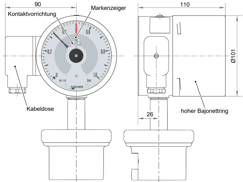
Abb. 23: Sicherheitsgehäuse
