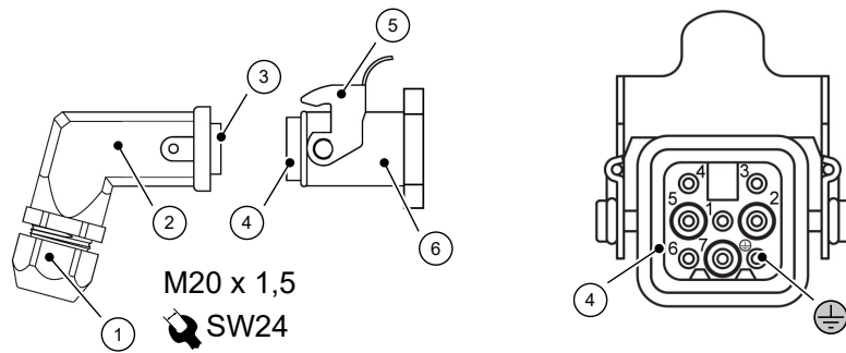
Abb. 8: HAN 7D
