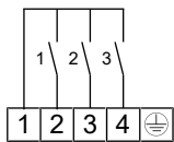
Abb. 9: Kontakte
