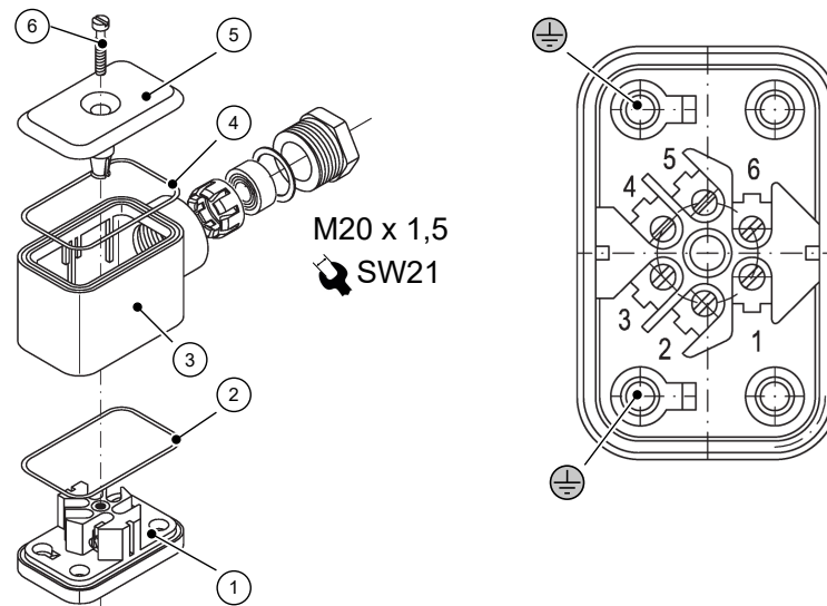
Abb. 7: Kabeldose
