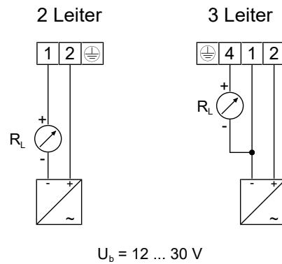
Abb. 11: Anschluss Drehwinkelgeber
