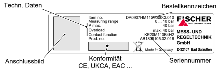
Abb. 4: Typenschild
