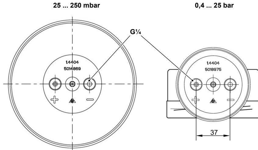
Abb. 19: Prozessanschluss
