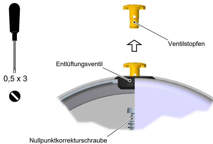
Abb. 13: Nullpunktkorrektur
