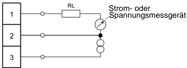
Abb. 6 Nullpunktjustierung (Dreileiter-Anschluss)
