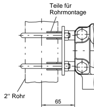
Zubehör: Montagesatz für 2"-Rohre DZ10
