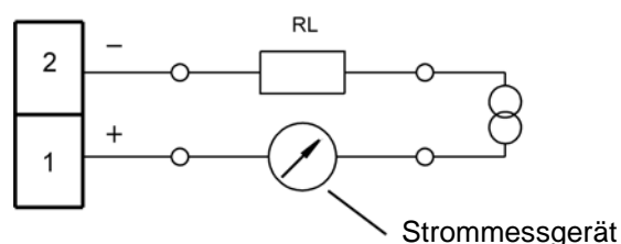
Abb. 5 Nullpunktjustierung (Zweileiter-Anschluss)
