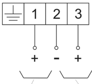
Abb. 3 Dreileiter-Anschluss
