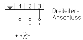
Dreileiter-Anschluss bei Geräten mit LCD
