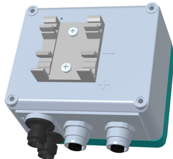
Tragschienenmontage
