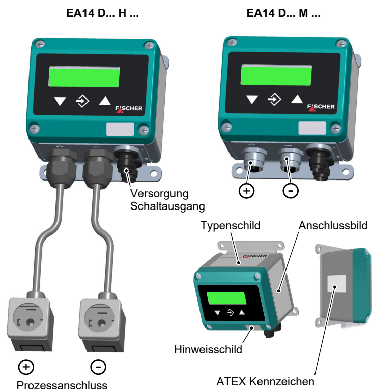
Abb. 2: Geräteausführungen
