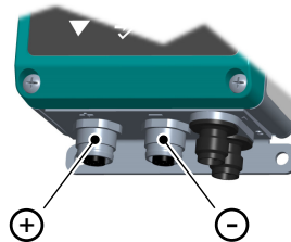
Abb. 5: Prozessanschluss
