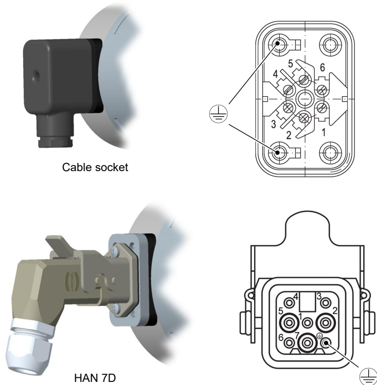
Fig. 21: Cable socket
