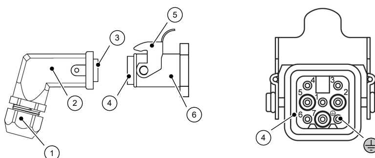
Fig. 13: HAN connector
