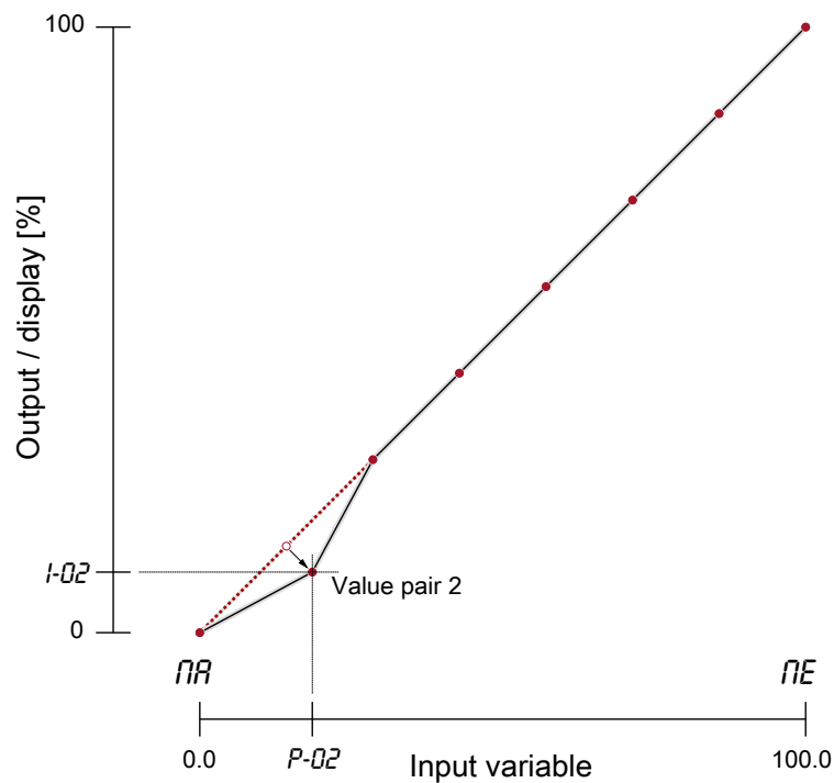
Fig. 10: Table function
