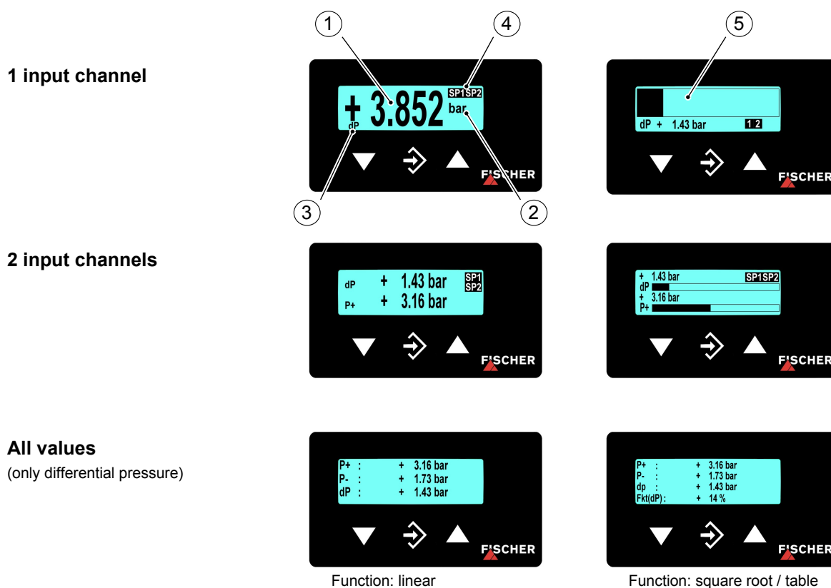
Fig. 10: LC display
