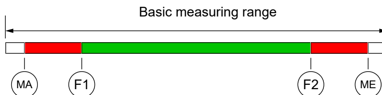
Fig. 16: Function Auto1
