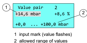
Fig. 14: Value pair
