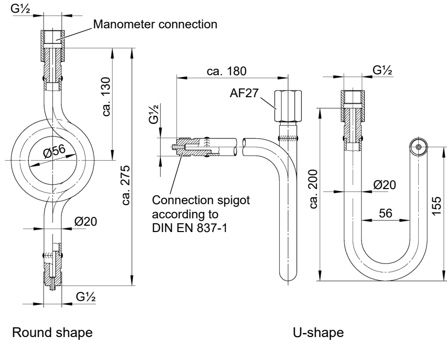
Fig. 6: Siphon MZ1###
