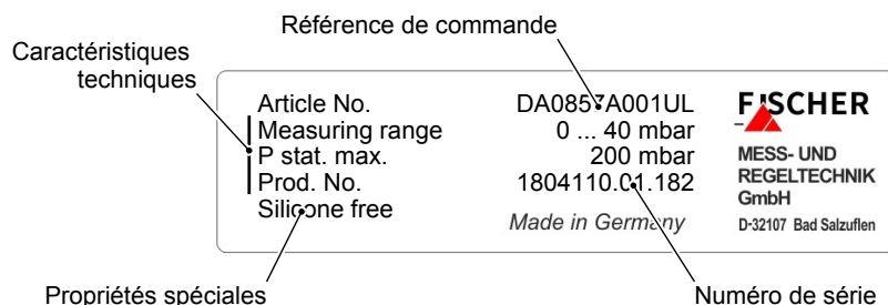
Fig. 3: Plaque signalétique
