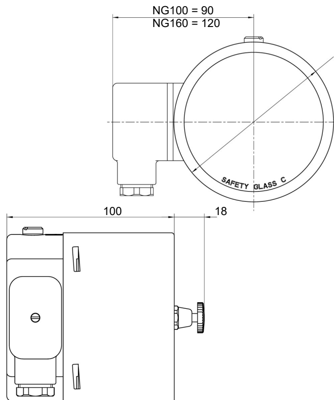
Рис. 24: Корпус с байонетным кольцом и кабельной коробкой
