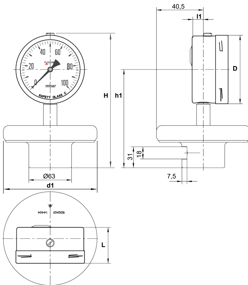
Рис. 17: Размерный чертеж 25... 250 мбар
