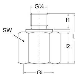
Рис. 22: Соединительная цапфа Gi
