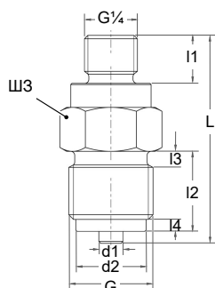
Рис. 20: Соединительная цапфа G
