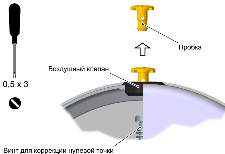
Рис. 13: Коррекция нулевой точки
