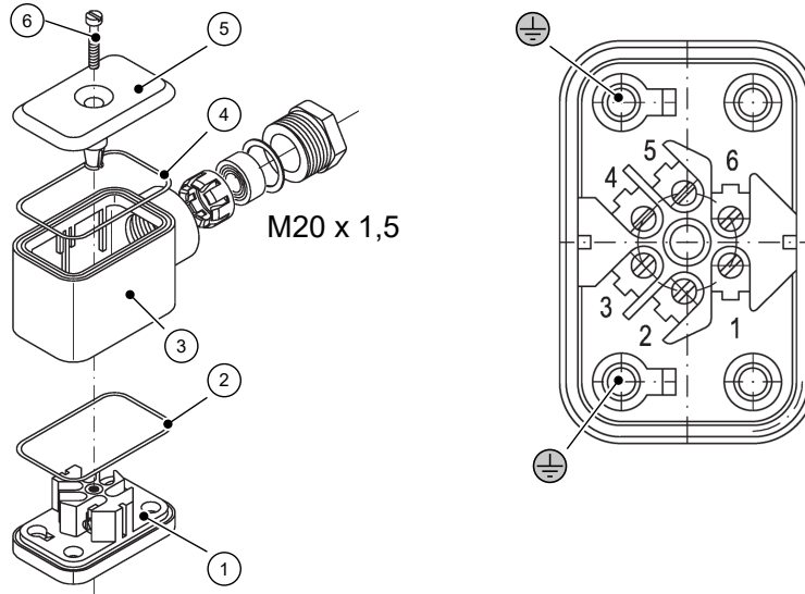
Рис. 8: Кабельная коробка
