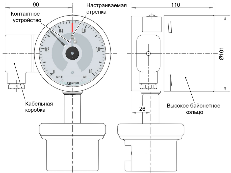
Рис. 23: Защитный кожух
