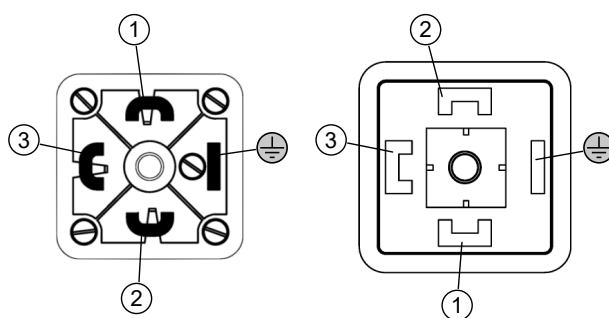
Штекер прибора Розетка кабельного разъема
