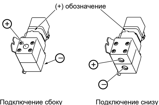
Рис. 5: Техническое подключение
