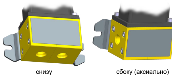
Рис. 2: Технологическое соединение
