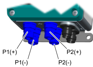
Рис. 5: Техническое подключение
