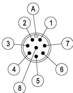
Рис. 25: M12 штекер 8-контактный
