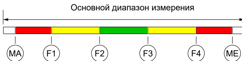
Рис. 21: Функция "Авто 2"
