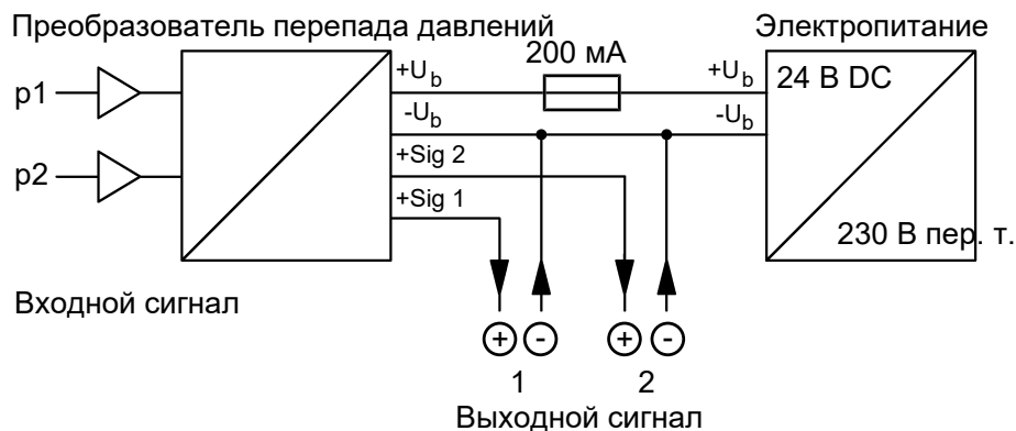
Рис. 6: Трехпроводное подключение
