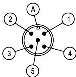
Рис. 23: M12 штекер 5-контактный
