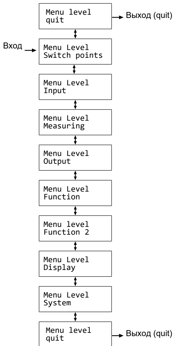
Рис. 16: Уровни меню
