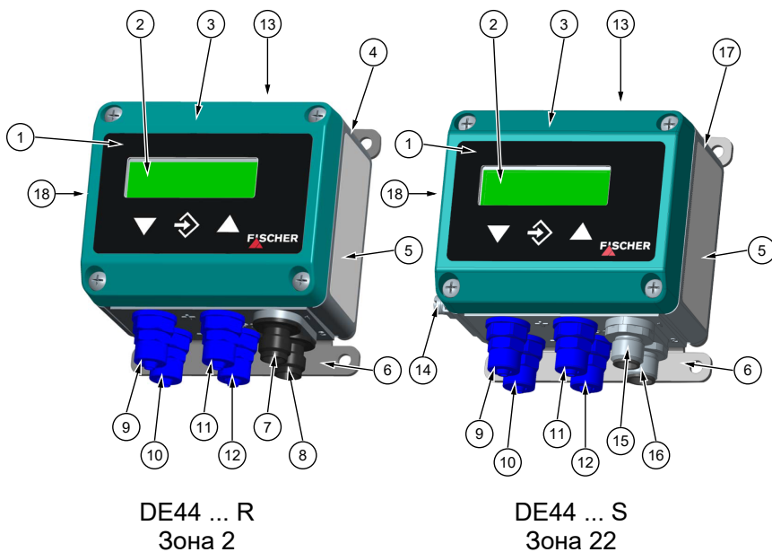
Рис. 3: Обзор DE44_LCD
