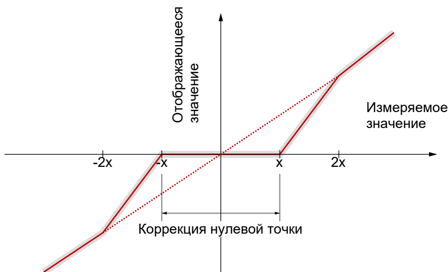
Рис. 17: Коррекция нулевой точки
