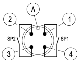
Рис. 24: Штекер M12 4-контактный
