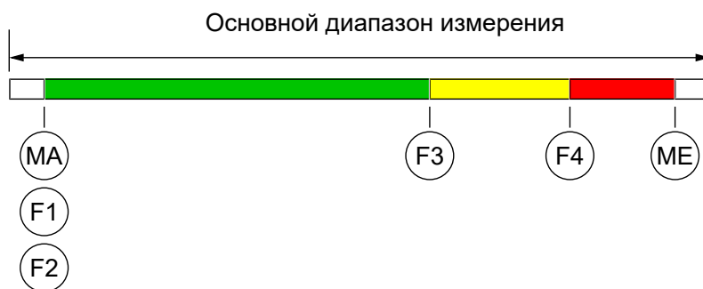
Рис. 22: Пример Авто 2
