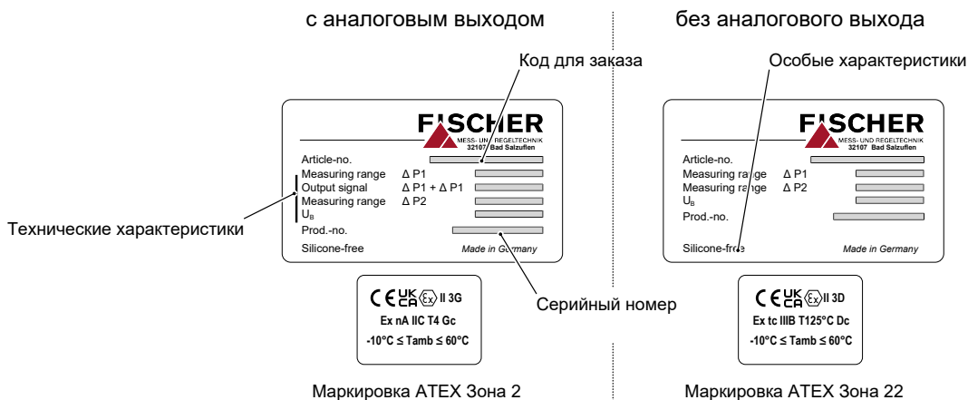
Рис. 4: DE44_LCD Паспортная табличка
