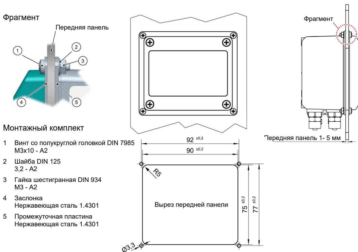
Рис. 29: Схема установки на передней панели
