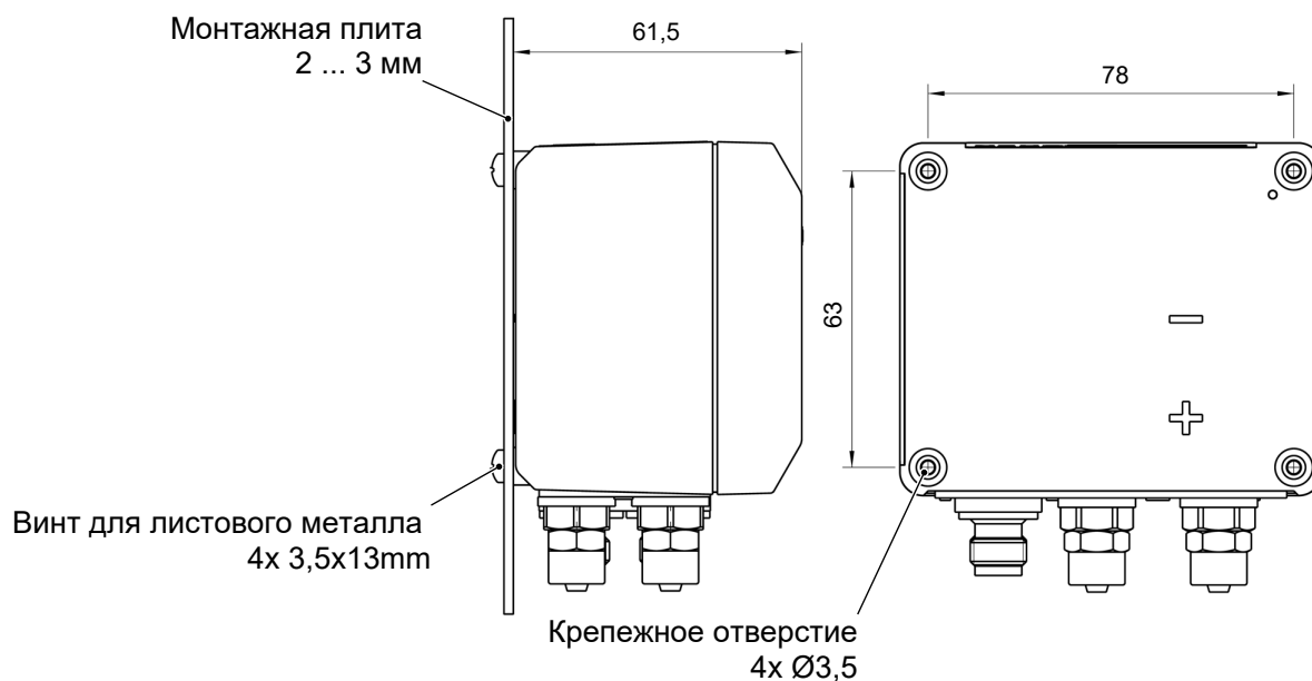
Рис. 28: Чертеж монтажной платы
