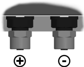
Рис. 3: Техническое подключение
