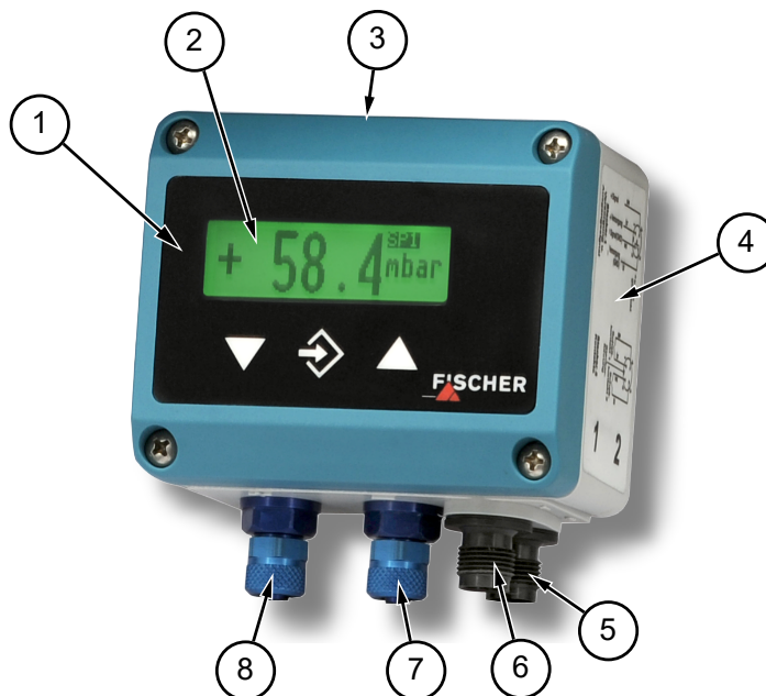
Рис. 1: Описание деталей
