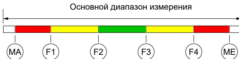
Рис. 16: Функция "авто 2"
