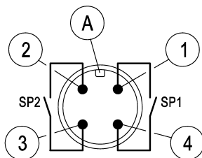
Рис. 18: Электроподключение DE45_LCD
