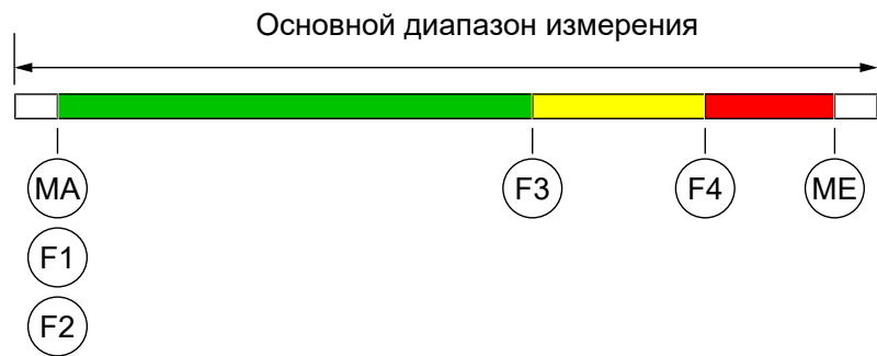
Рис. 17: Пример Авто 2
