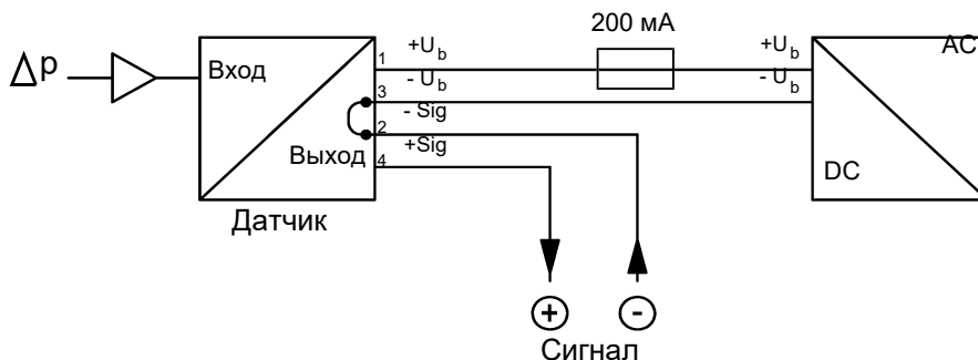
Рис. 4: Трехпроводное подключение с внутренним мостом
