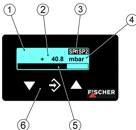
Рис. 8: ЖК-дисплей DE45
