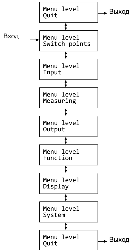
Рис. 11: Уровни меню
