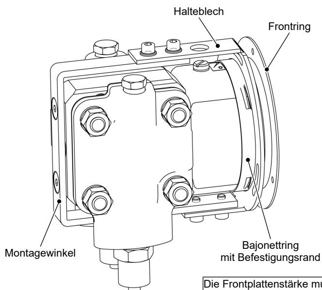
Abb. 15: Fronttafeleinbau mit Tafeleinbaugarnitur
