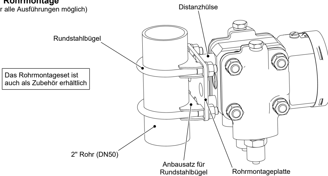
Abb. 13: Rohrmontage
