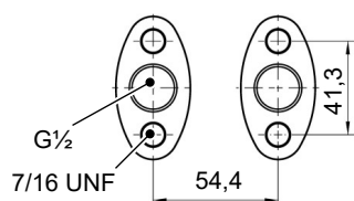
Abb. 14: Maßbild (Großes Messsystem Ø130)
