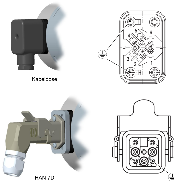
Abb. 11: Kabeldose
