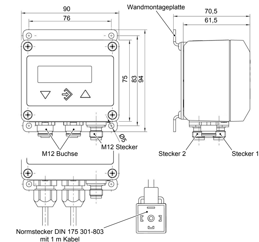
Abb. 4: Maßbild
