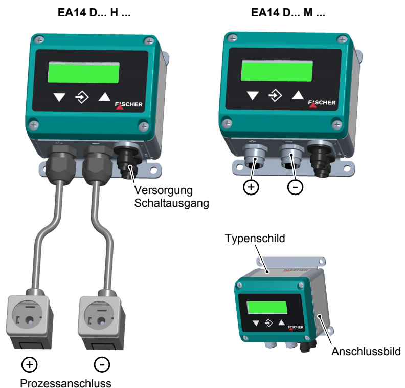
Abb. 1: Geräteausführungen
