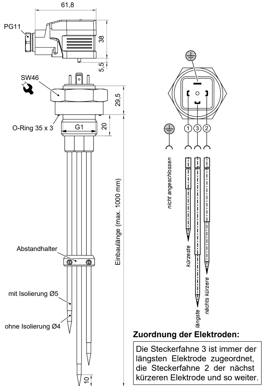
Abb. 3: Maßzeichnung
