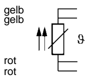
Einfach Pt100 4-Leiter-Schaltung
