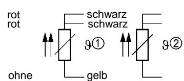
Doppel Pt100 3-Leiter-Schaltung
