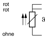
Einfach Pt100 3-Leiter-Schaltung
