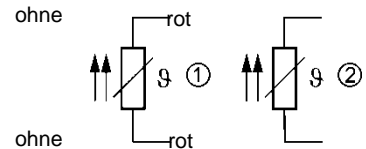
Doppel Pt100 2-Leiter-Schaltung
