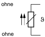
Einfach Pt100 2-Leiter-Schaltung
