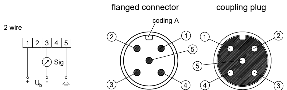
Fig. 7: M12 coupling plug DIN EN 61076-2-101
