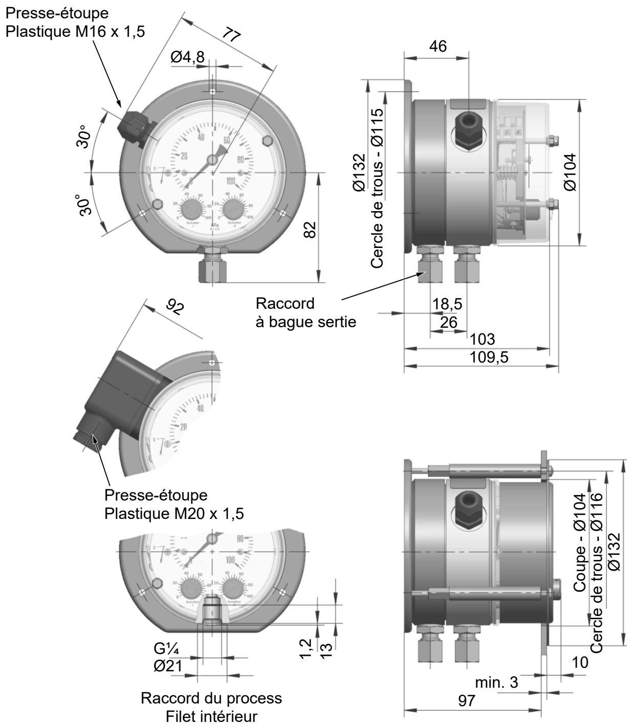
Fig. 8: Chambre de pression en acier inox (IP55)
