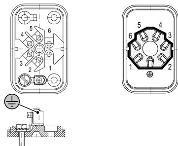
Fig. 5: Prise/fiche de câble
