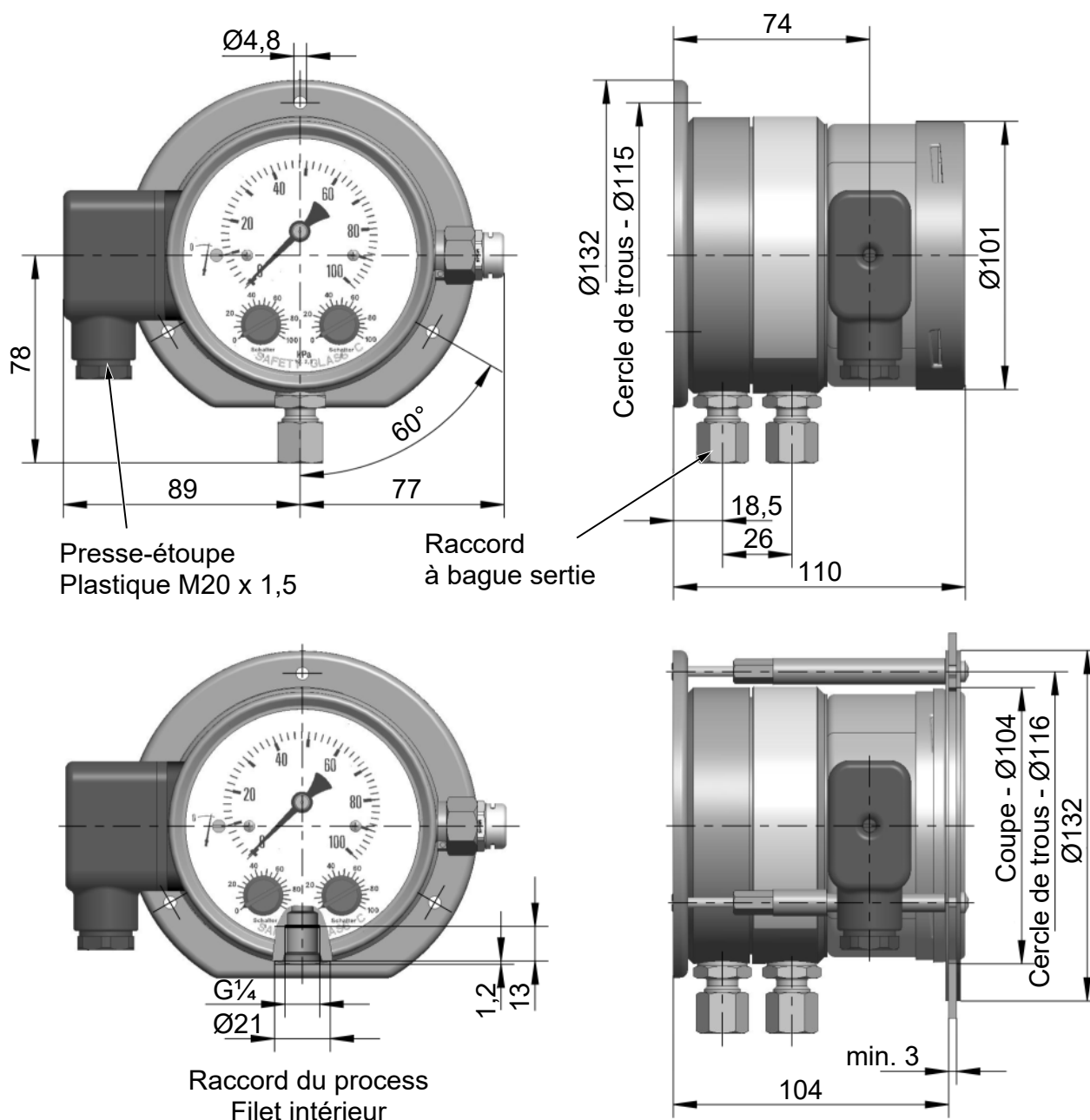
Fig. 9: Chambre de pression en acier inox (IP65)
