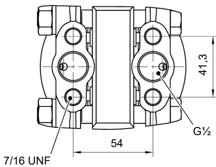
Рис. 8: Схема установки (малая измерительная система Ø 75)
