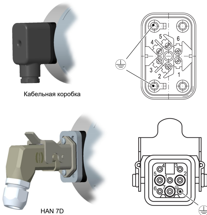
Рис. 7: Кабельная коробка
