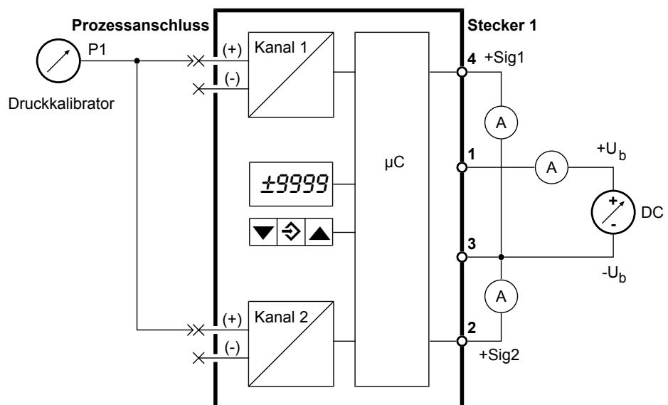
Abb. 1: Funktionstest
