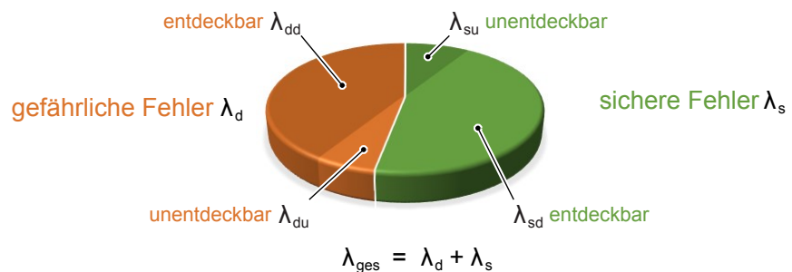
Abb. 5: Fehlerraten
