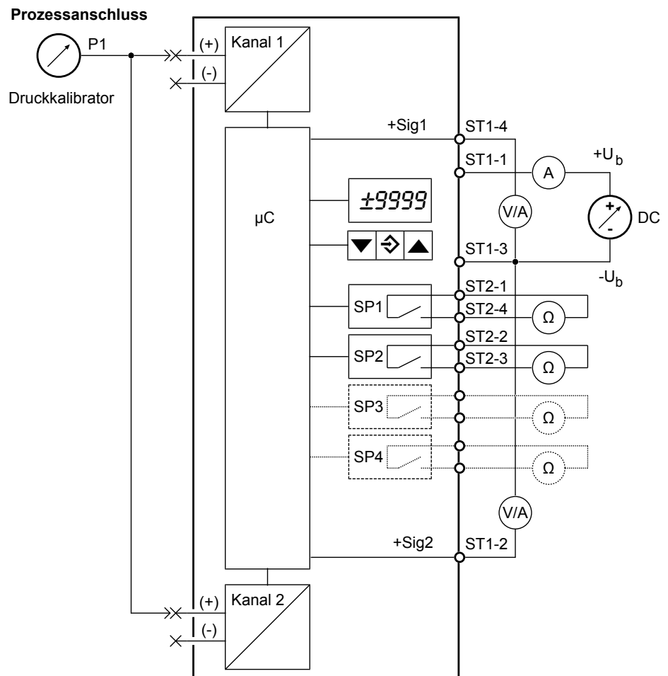
Abb. 4: Funktionstest
