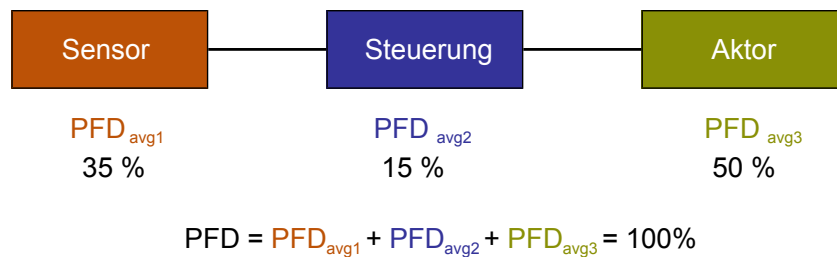
Abb. 2: PFD Aufteilung
