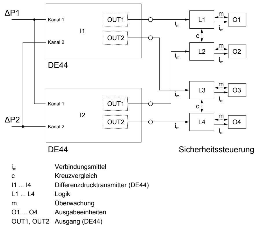
Abb. 3: Anschlussschema
