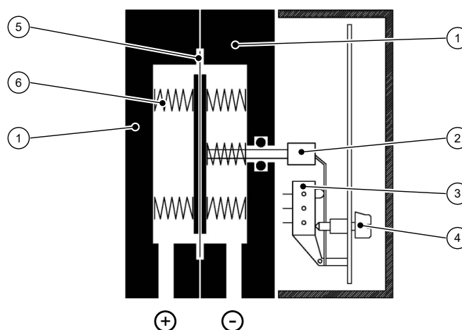
Abb. 1: Funktionsbild
