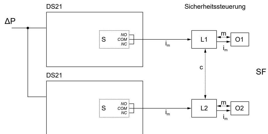
Abb. 3: Architektur 1oo2
