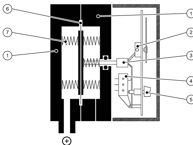
Abb. 1: Funktionsbild
