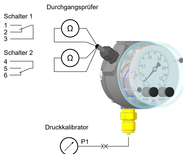
Abb. 4: Funktionstest
