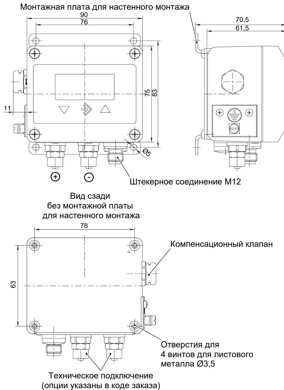
Рис. 4: Размерный чертеж
