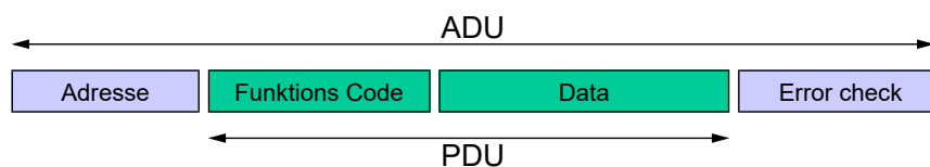
Abb. 4: MODBUS Frame
